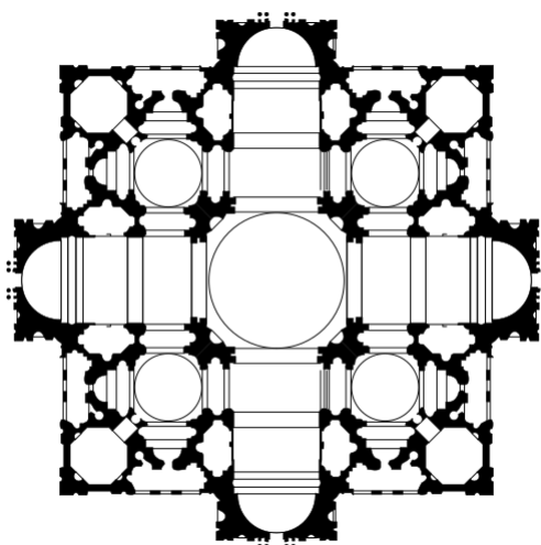
План Донатто Браманте собора Святого Петра
